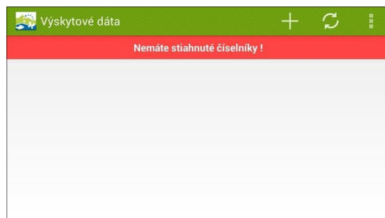
Obrázok 3: Nezosynchronizované číselníky
