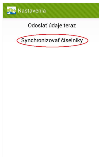
Obrázok 4: Synchronizácia číselníkov
