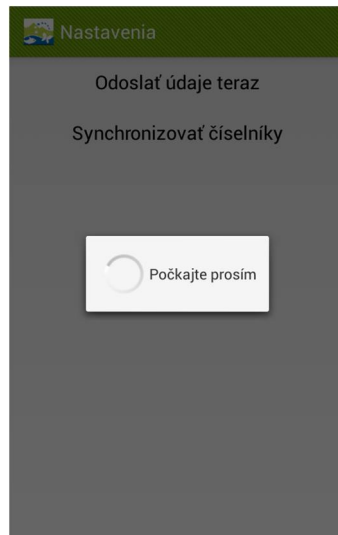
Obrázok 5: Synchronizácia číselníkov
