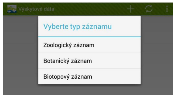
Obrázok 7: typ záznamu
